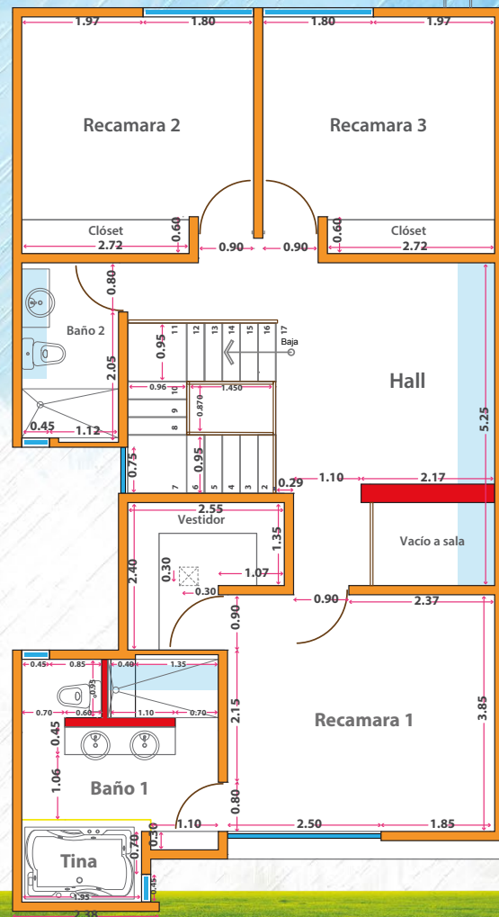
PLANTA ARQUITECTONICA ALTA
