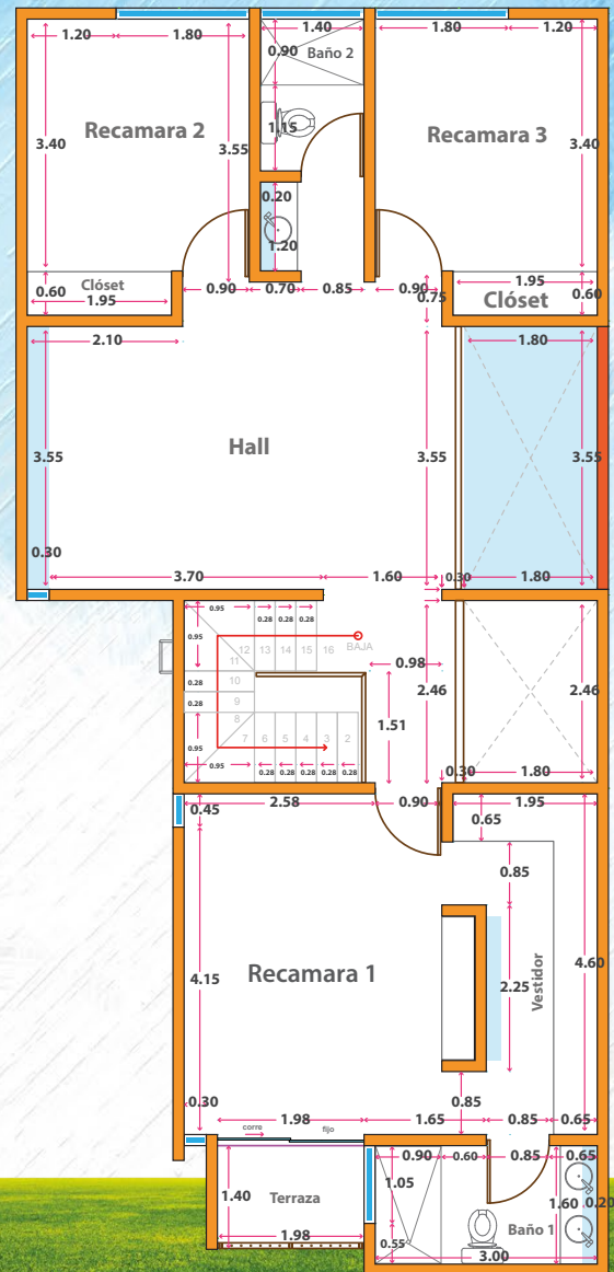
PLANTA ARQUITECTONICA ALTA
